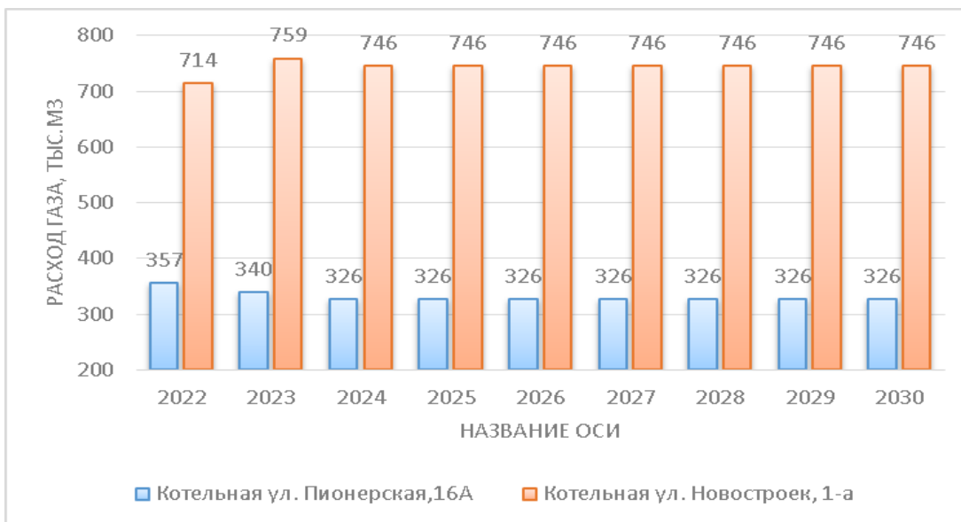
Рисунок 8.1.1 - Динамика потребления газа котельных
